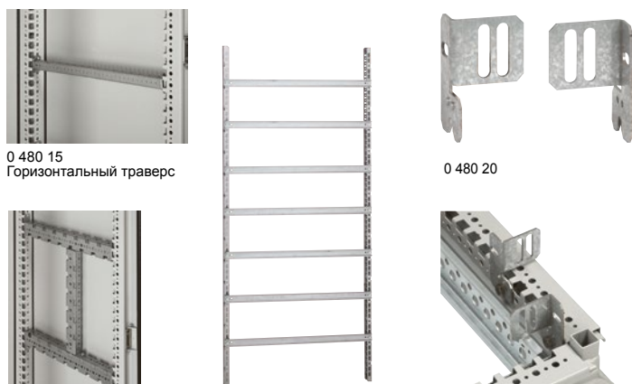
0 480 15 Горизонтальный траверс
